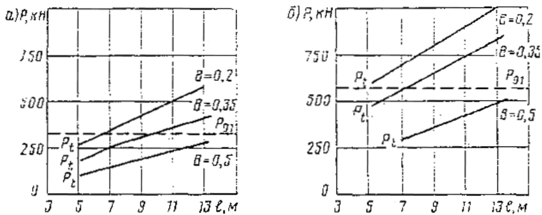
Рис. 2. Несущая способность железобетонных свай сечением 22x22 см (а) и 35X35 см (б) в суглинках с различными коэффициентами консистенции B
