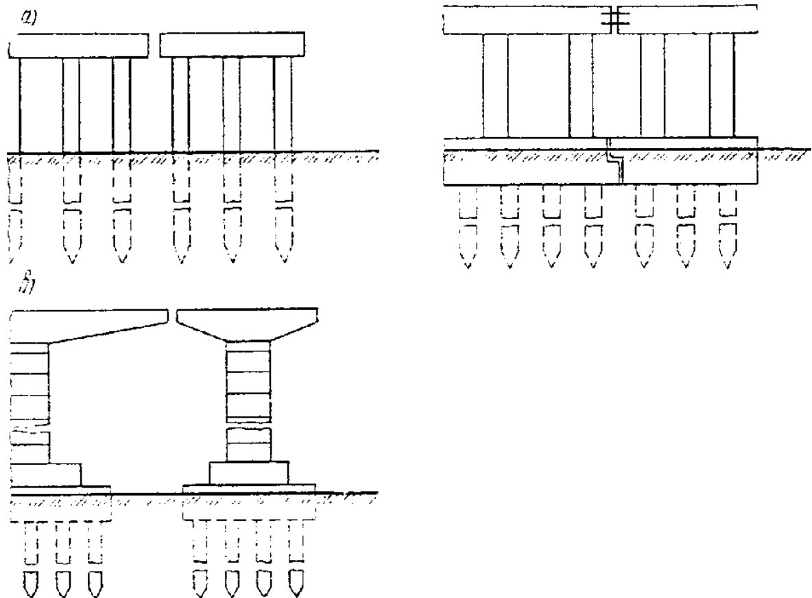
Рис. 3.19. Схемы уширения промежуточных опор с развитием фундамента опор:
