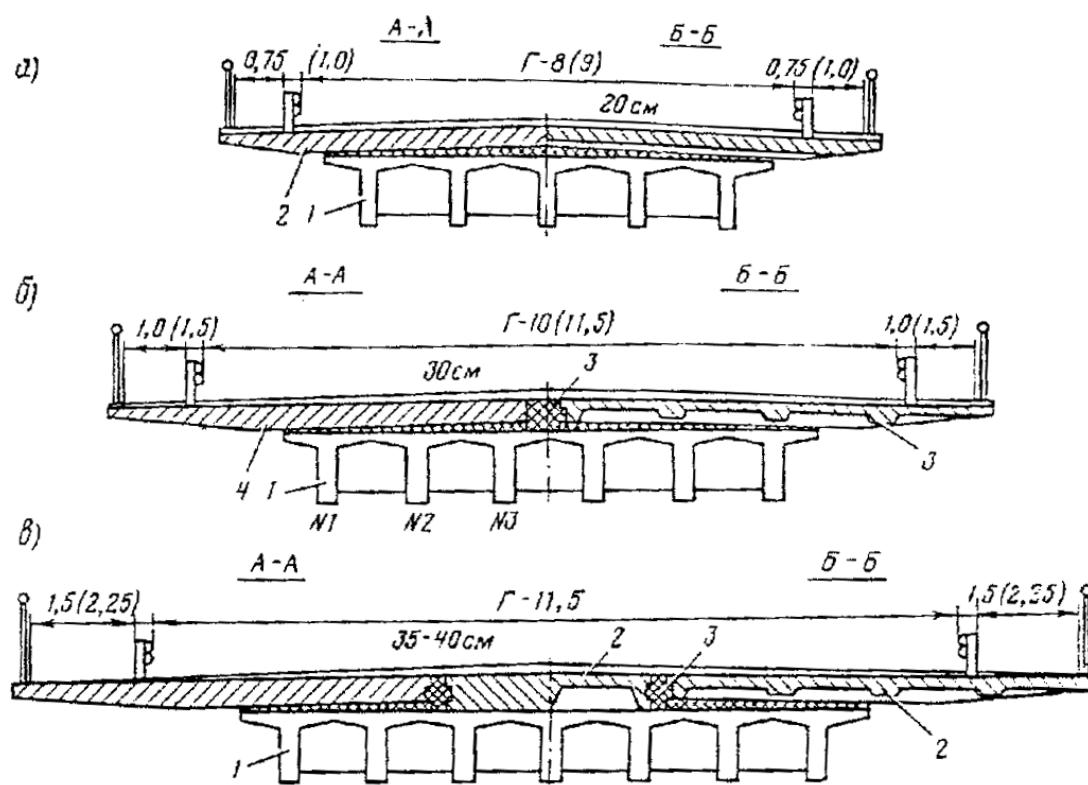
Рис. 3.4. Схемы уширения сборной (а) и сборно-моноклитной (б, в) накладной плитой:
