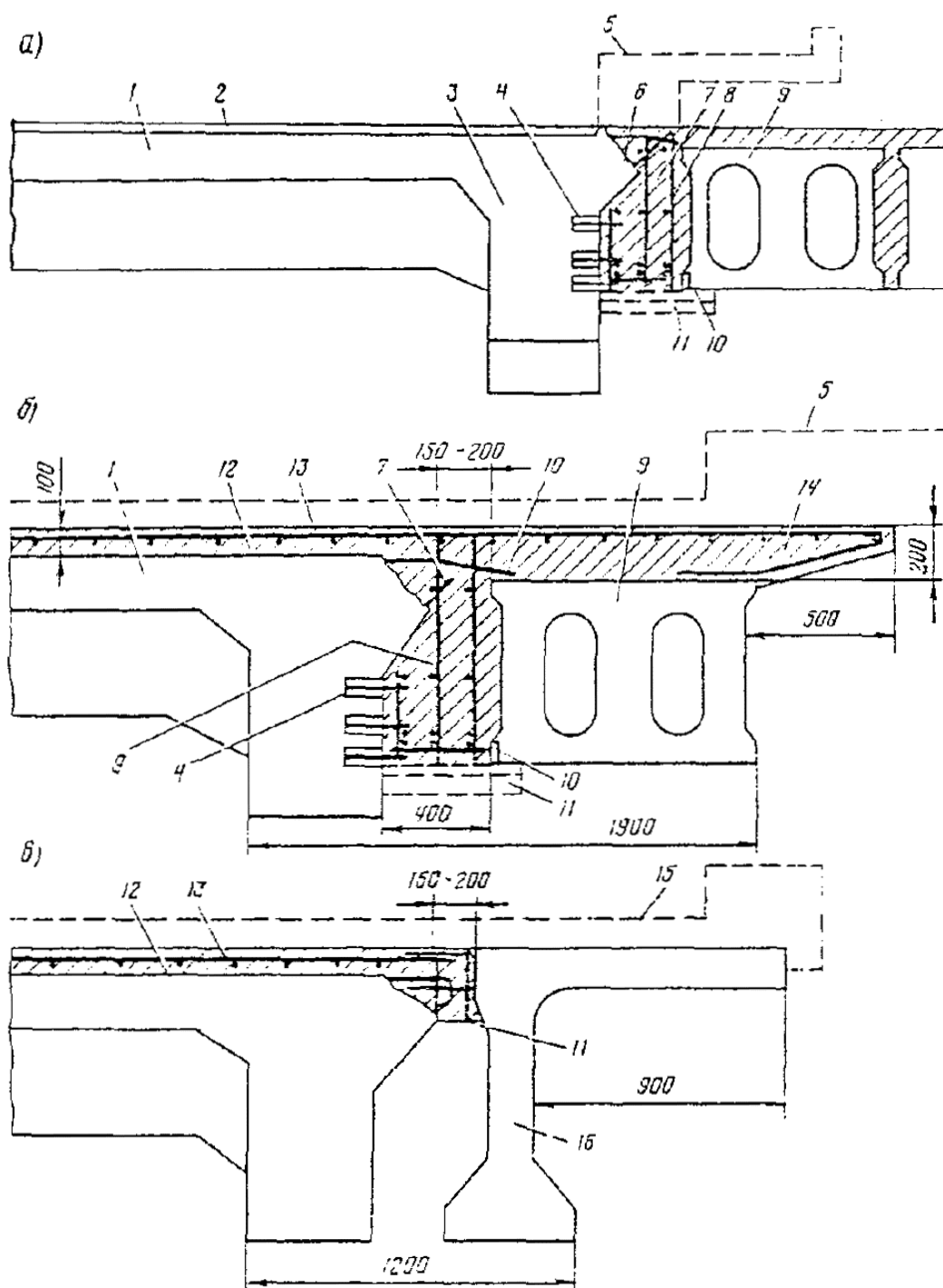
Рис. 4.9. Узел объединения монолитного ребристого пролетного строения с приставляемыми плитами (а, б) и балкой (в):
