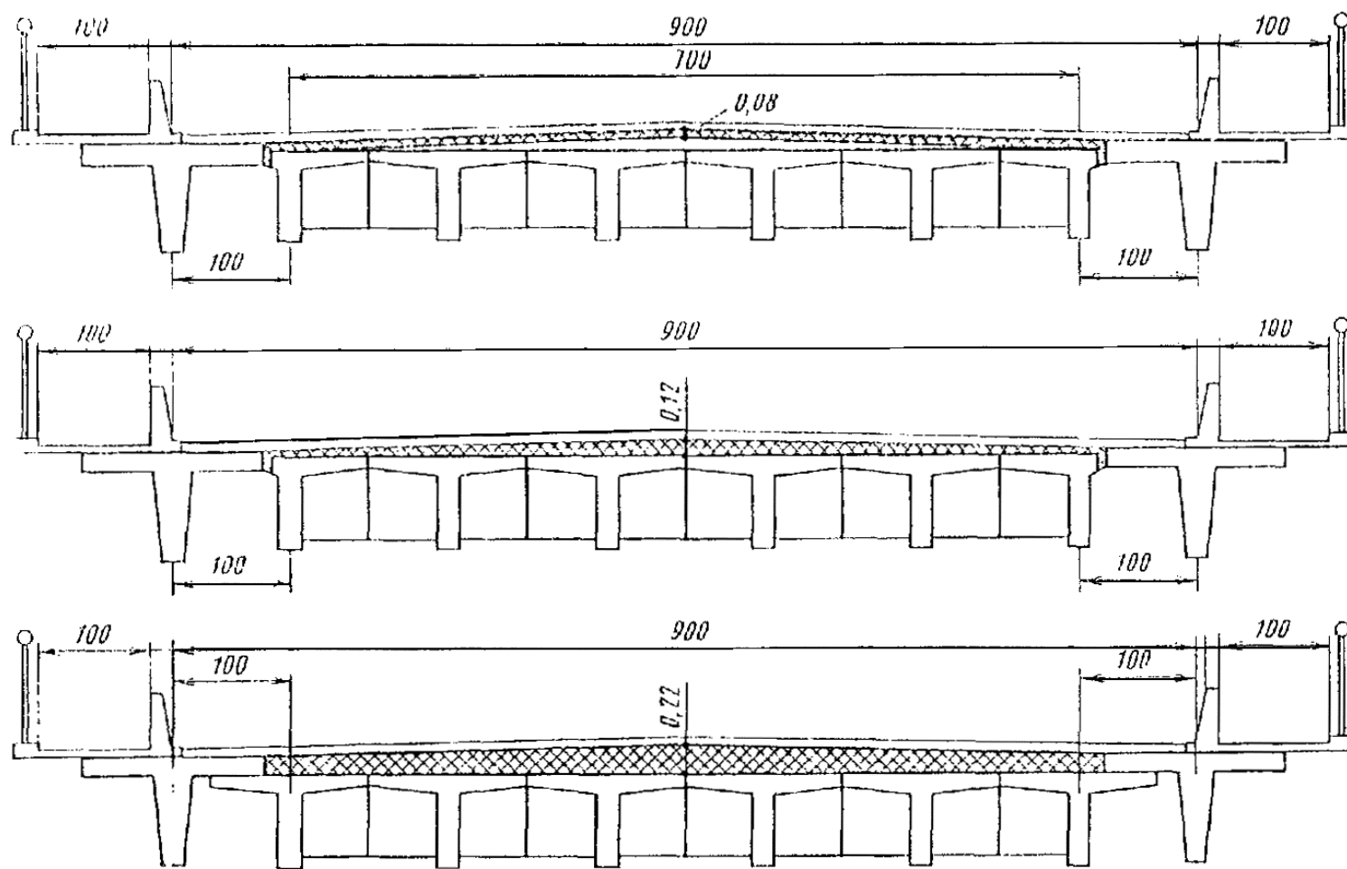
Рис. 6.7. Уширение пролетных строений из балок по типовому проекту 56 с помощью приближенных на 1 м балок с габарита Г-7+1X0,75 до Г-9+2X1,0 м
