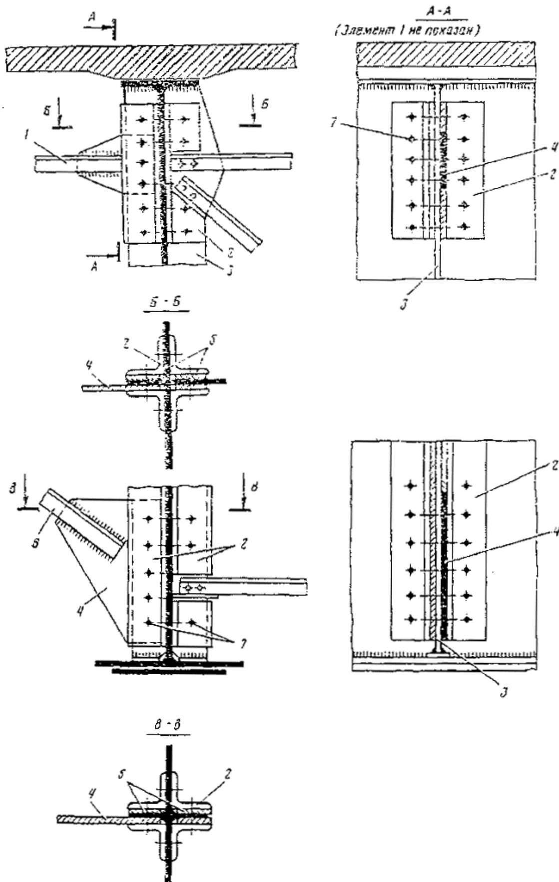
Рис. 4.8. Узел крепления поддерживающих консолей к ребру жесткости балки:
