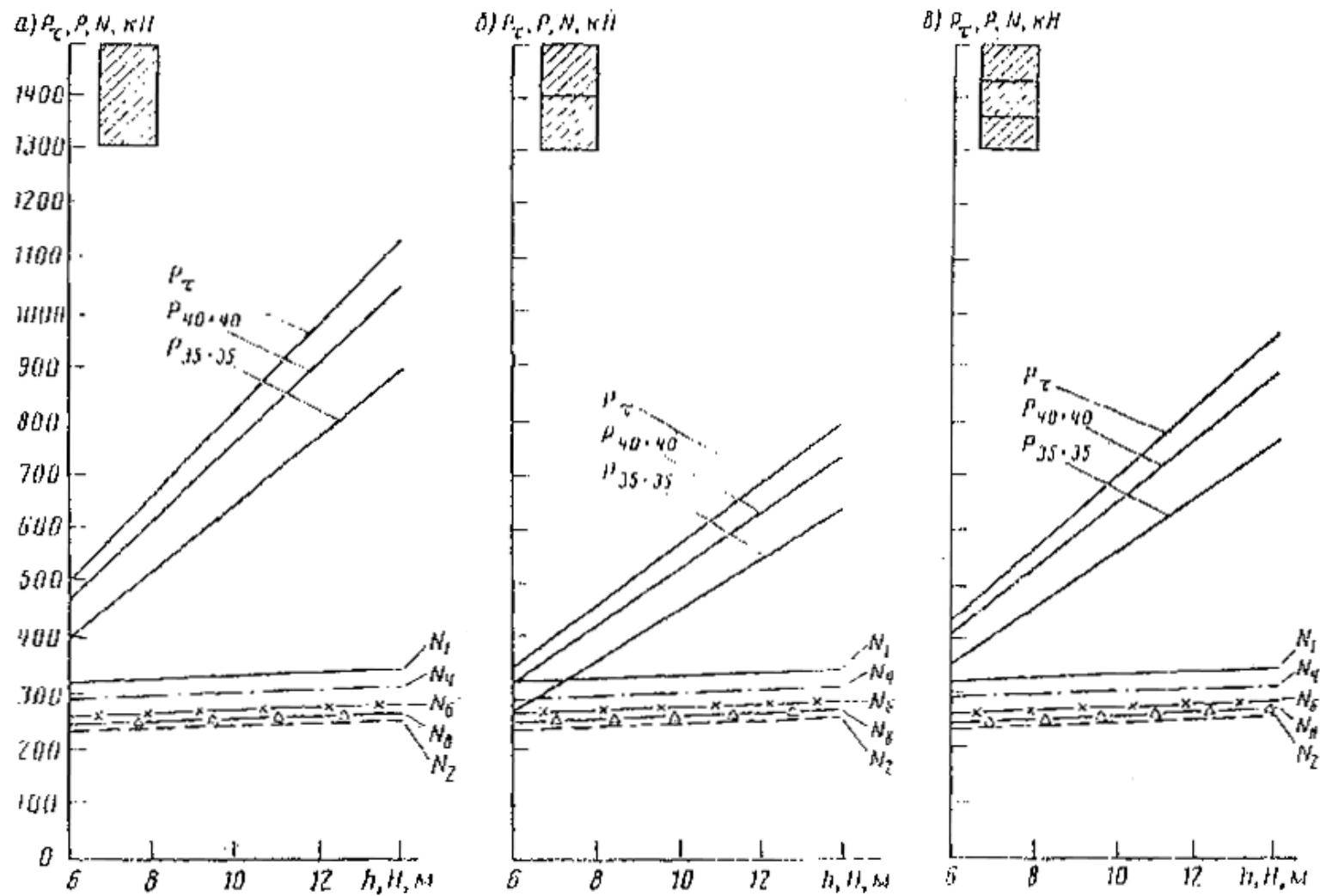
Рис. 5. Расчетные усилия в сваях устоя моста с длиной пролетных строений 11,36 м
