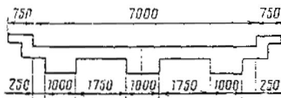
Рис. 7. Поперечное сечение, плитно-ребристого пролетного строения
