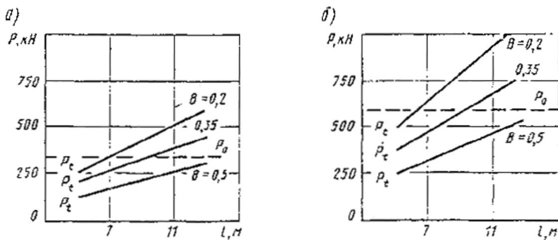
Рис. 3. Несущая способность железобетонных свай сечением 22x22 см (а) и 35x35 см (б) в глинах с различными коэффициентами консистенции B
