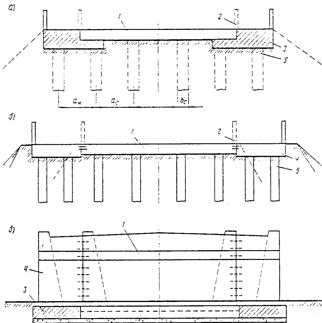
Рис. 3.20. Схемы уширения устоев:
