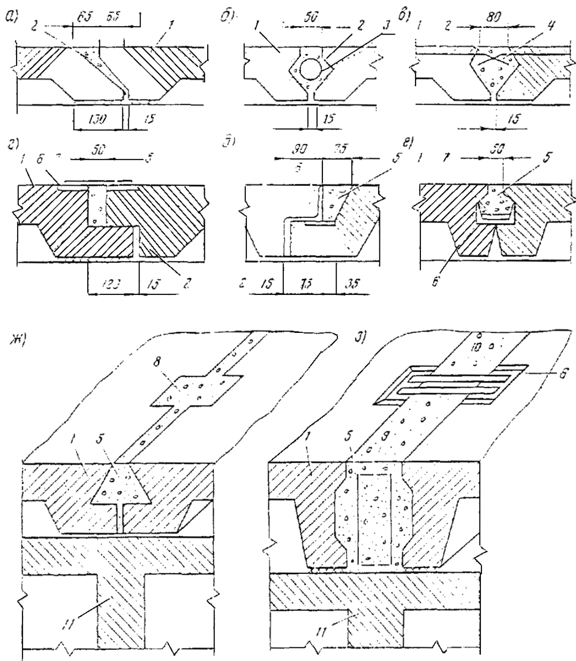
Рис 4.6. Стыки сборных блоков накладной плиты:
