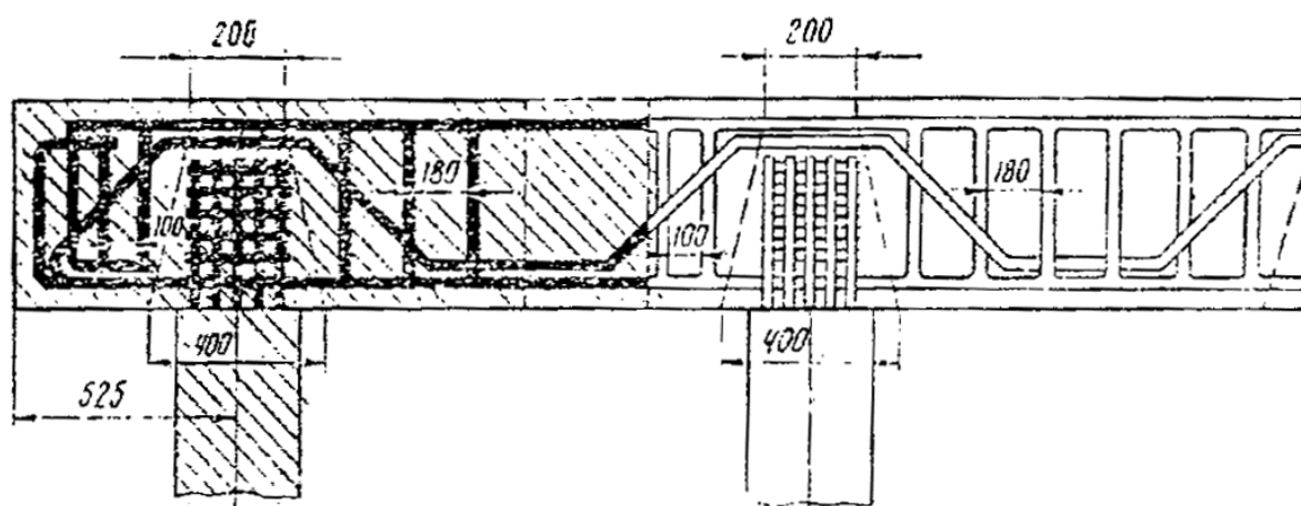
Рис. 6.12. Уширенная насадка опоры
