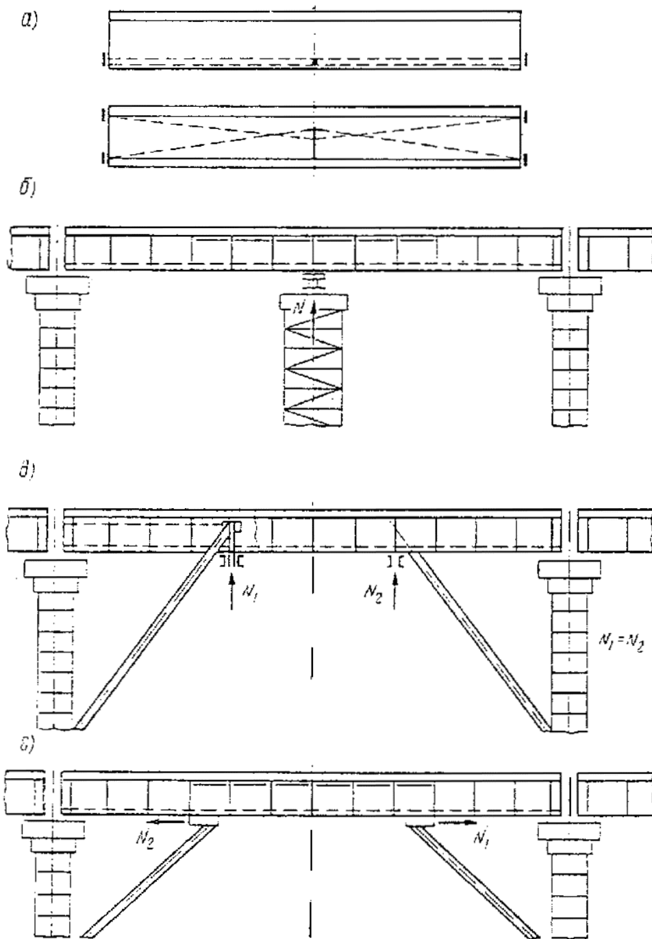
Рис. 5.1. Методы регулирования усилий:
