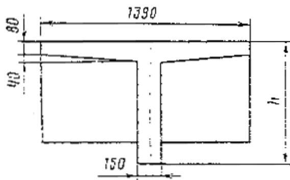
Рис. 1. Поперечное сечение балки ребристого пролетного строения по ТП (1)
