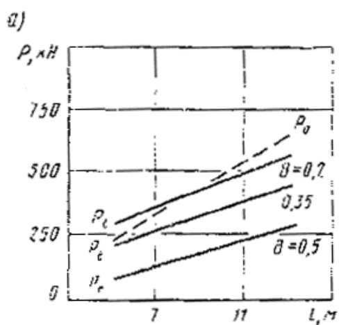
Рис. 6. Несущая способность деревянных свай d=28 \text{ см} (а) и d=40 \text{ см} (б) в сухих глинах с различными коэффициентами консистенции B
