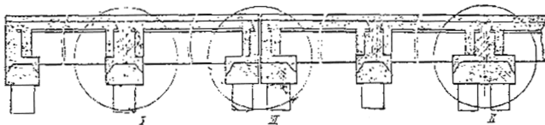
Рис. 6.3. Схема секционного моста после реконструкции
