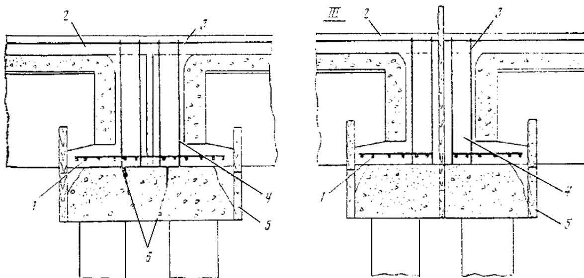
Рис. 6.5. Узлы II и III (см. рис. 6.3 ):
