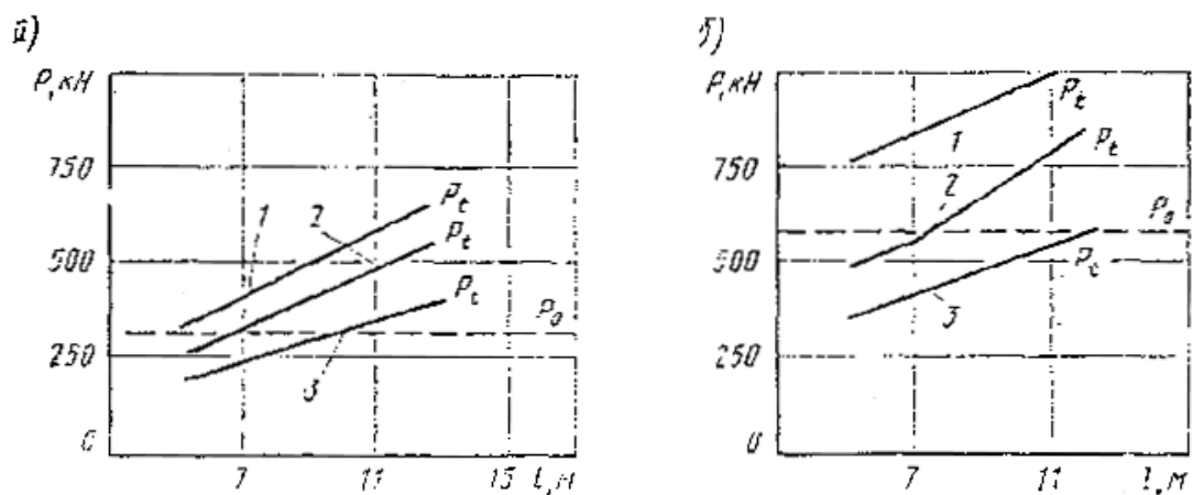
Рис. 1. Несущая способность железобетонных свай сечением 22x22 см (а) и 35X35 см (б) в песчаных грунтах:
