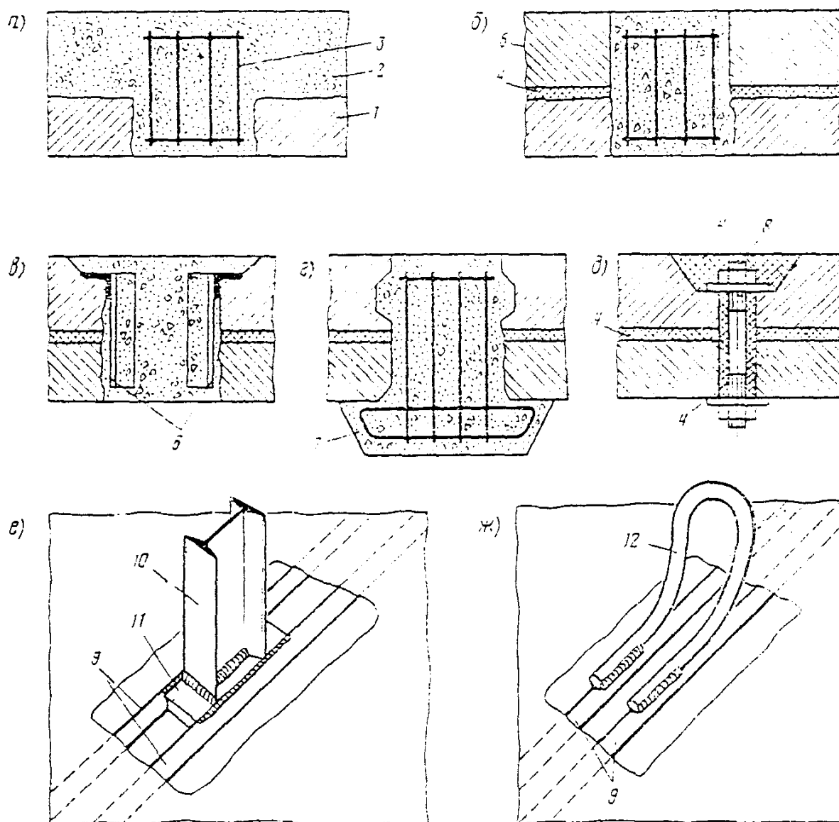
Рис. 4.5. Узлы объединения накладной плиты с существующими балками:
