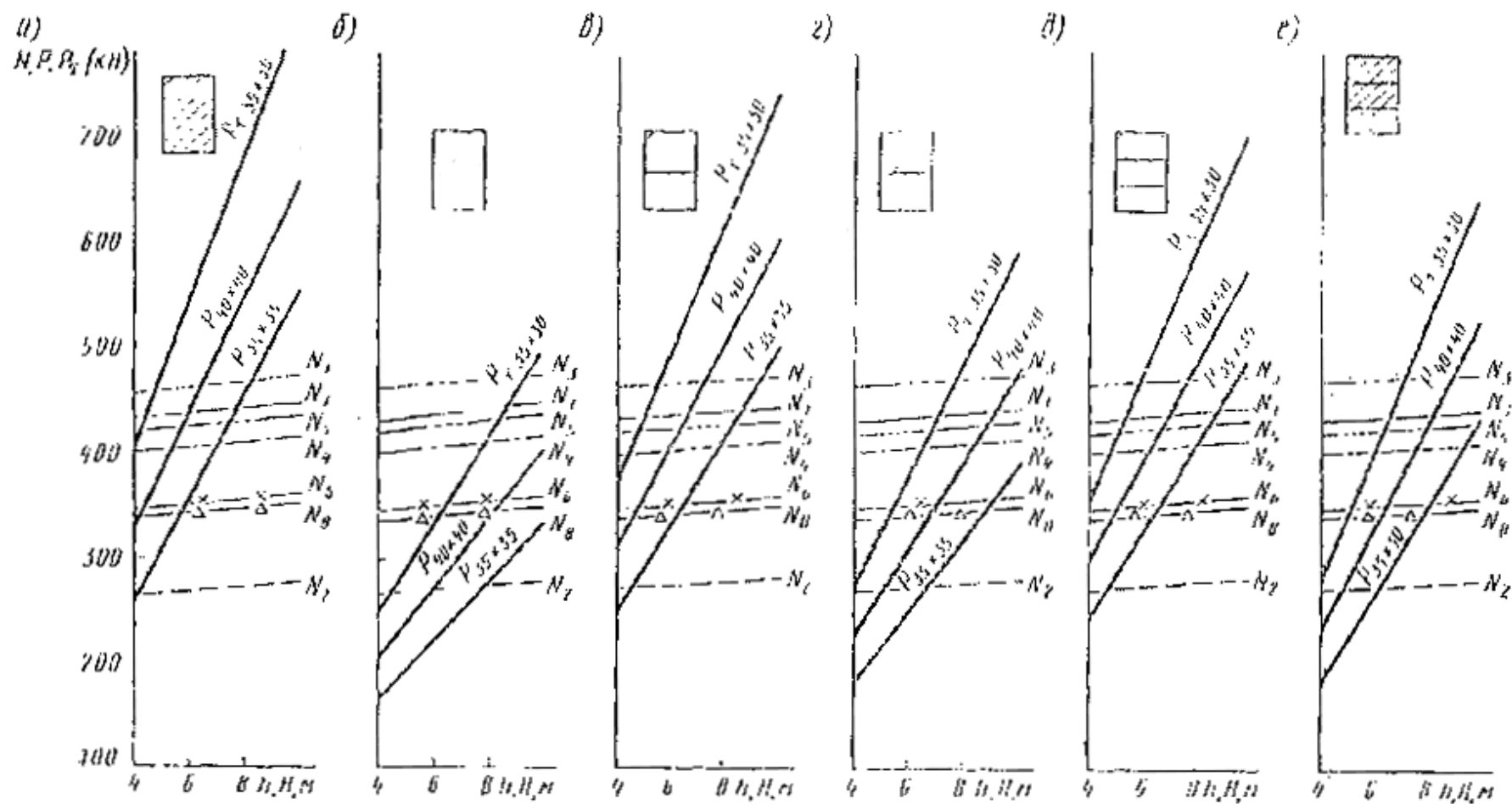
Рис. 4. Расчетные усилия N_i , приходящиеся на голову сваи при различном их погружении под промежуточной опорой моста с длиной пролетных строений 16,76 м
