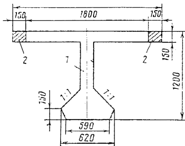
Рис. 4. Поперечное сечение элемента пролетного строения из унифицированных балок по ТП (3):
