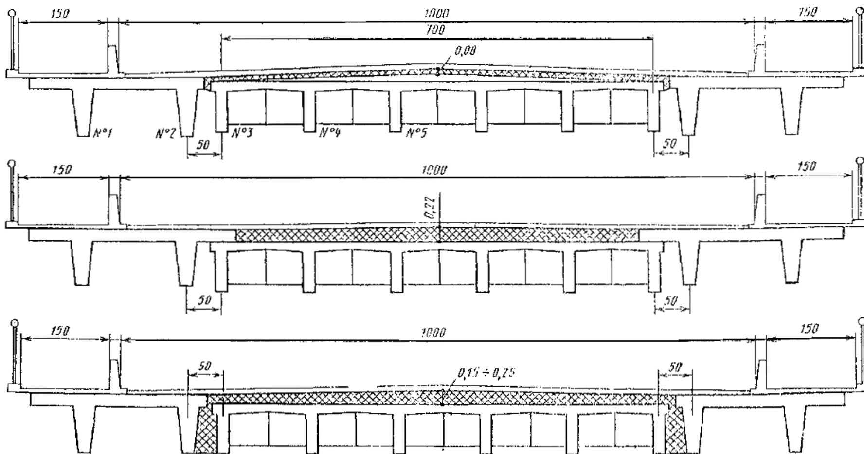
Рис. 6.8. Уширение пролетных строений из балок по типовому проекту 56 с помощью вплотную приставляемых с двух сторон балок с габарита Г-7+2X0,75 до Г-10+2X1,0 м
