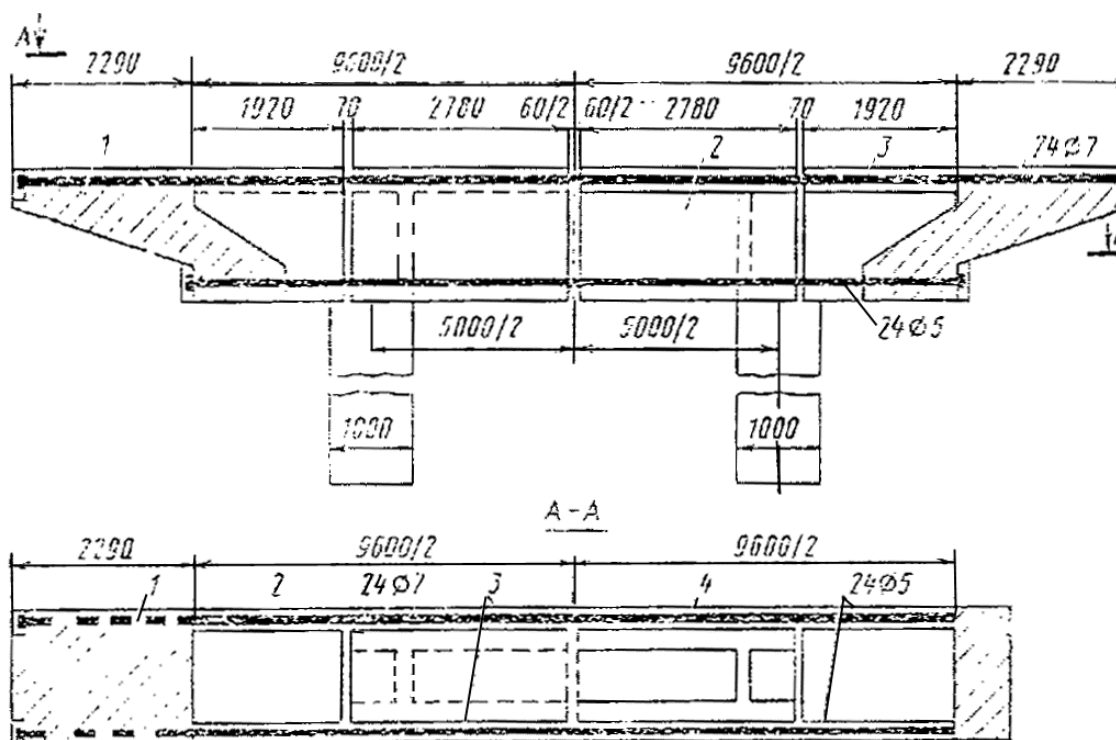
Рис. 6.13. Расположение дополнительных железобетонных блоков и напрягаемой арматуры в уширенной опоре:
