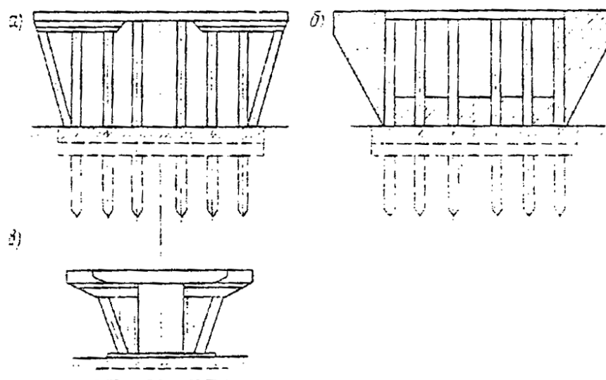
Рис. 3.17. Схемы уширения стоечных (а, б) и столбчатых (в) опор за счет развития их тела
