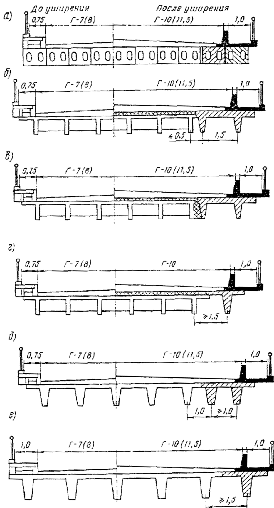
Рис. 3.6. Схемы увеличения габарита добавлением балок пролетных строений, требующих уширения тела опоры (группа В, б)
