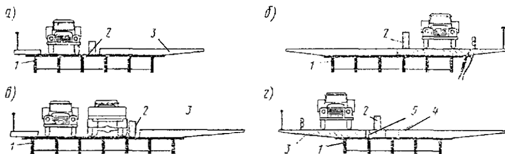
Рис. 5.2. Схемы организации движения по мосту, ушряемому сборной накладной плитой:
