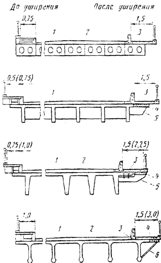
Рис. 3.1. Схемы увеличения ширины тротуаров (группа А):
