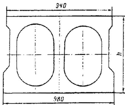
Рис. 2. Поперечное сечение пустотной плиты длиной 12, 15, 18 м по ТП (2, 4)
