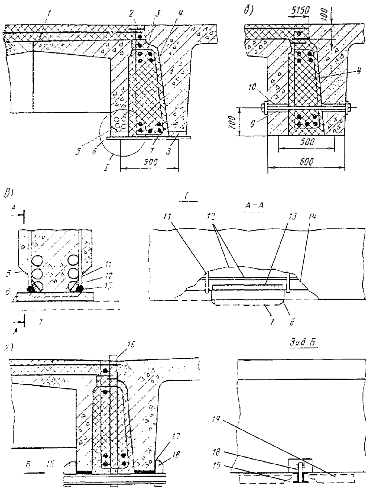
Рис. 4.4. Схема стыковки балок с помощью накладок (а, в), болтов (б), захватов (г):
