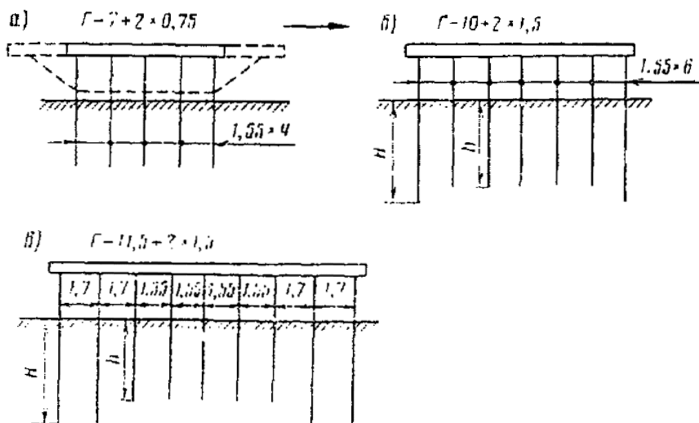
Рис. 2. Схемы уширения промежуточных опор:
