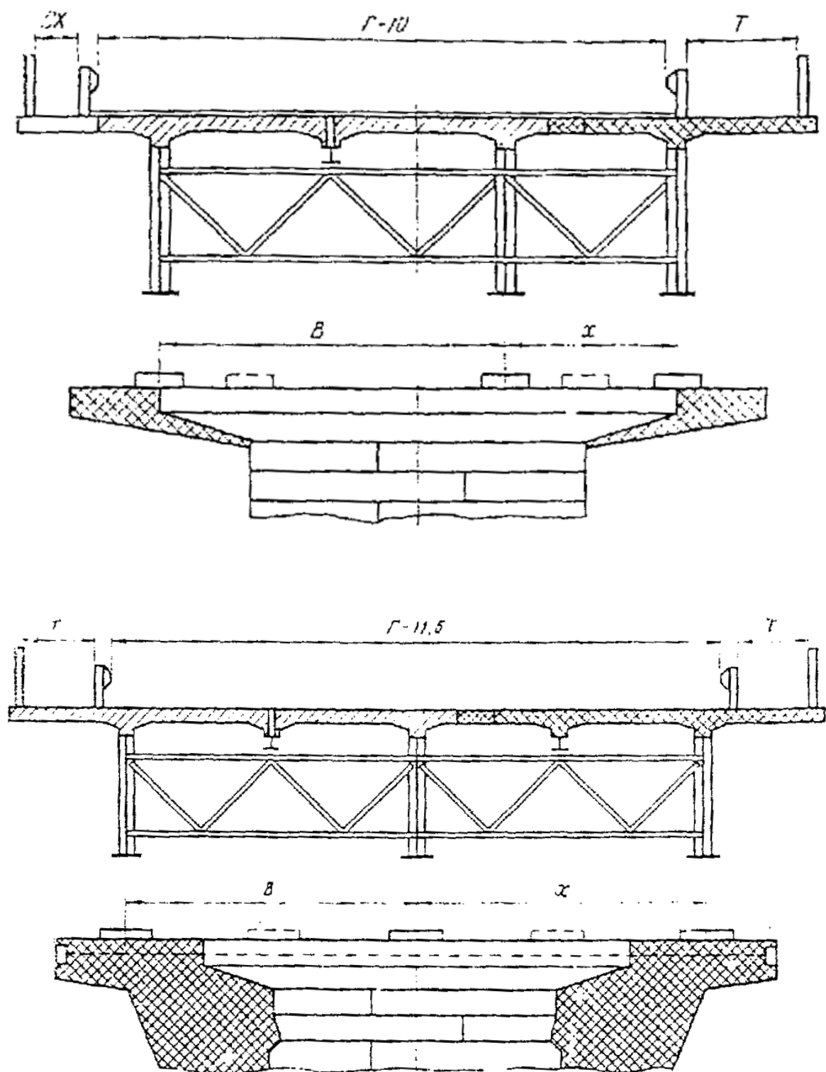
Рис. 3.15. Схемы уширения сталежелезобетонных пролетных строений добавлением новых балок
