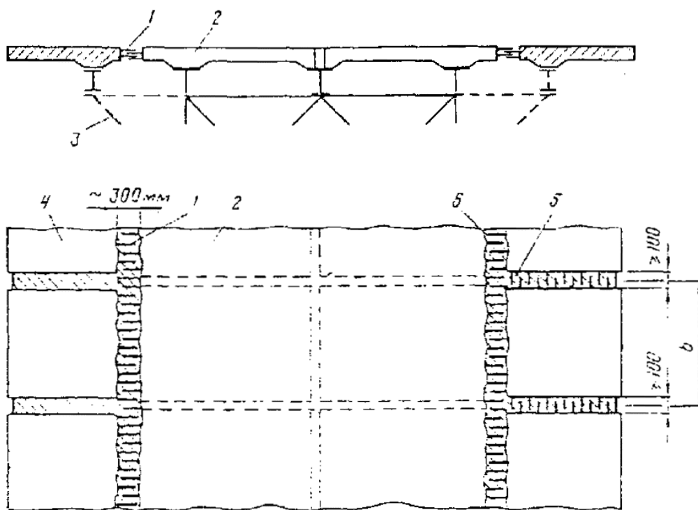
Рис. 4.7. Схема расположения элементов уширения:
