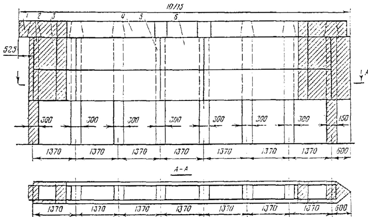
Рис. 6.10. Вид свайной опоры после уширения:
